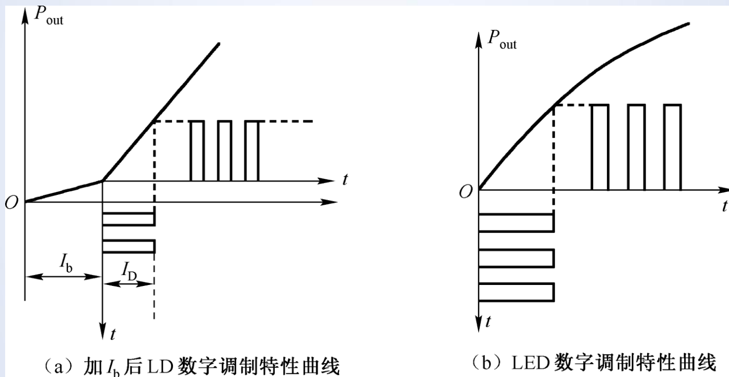
图3-10 数字调制特性
